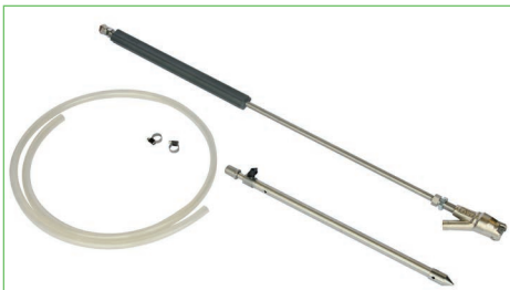
Gritstraallans van 900 mm met vlakstraalsproeier, snelkoppeling en aanzuigbuis geschikt voor werkdruk ≤ 500 bar code: 1.258.229.00xxx code: 1.258.229.15xxx
